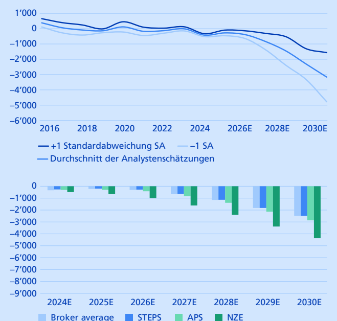
Abbildung 11: Das Kupfer-Gleichgewicht.
